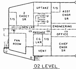
O2 LEVEL
