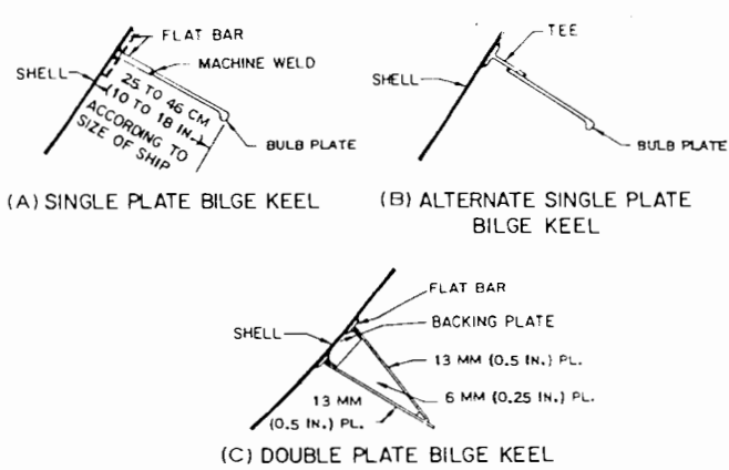
Fig. 82 Bilge keels
