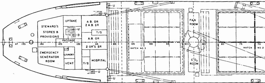
O1 LEVEL
