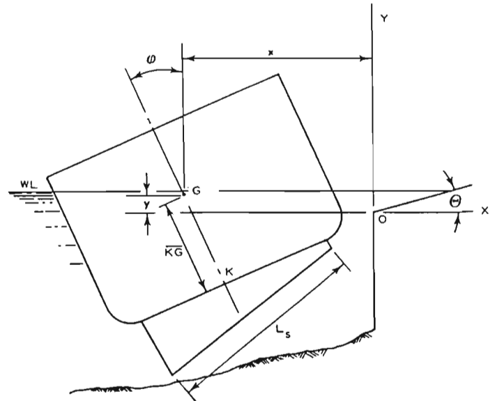
Fig. 28 Phase 4—dropping
