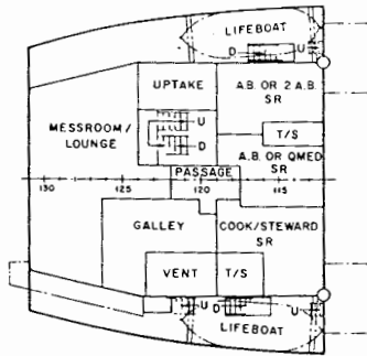
O1 LEVEL
